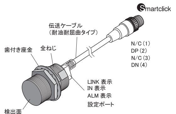
BS-K1117M-M18-3012の例
