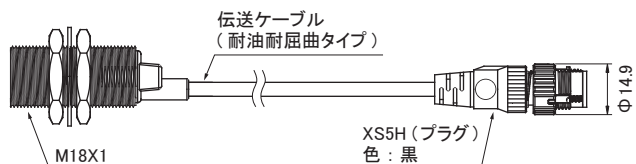
BS-K1117M-M18-3012 の例
